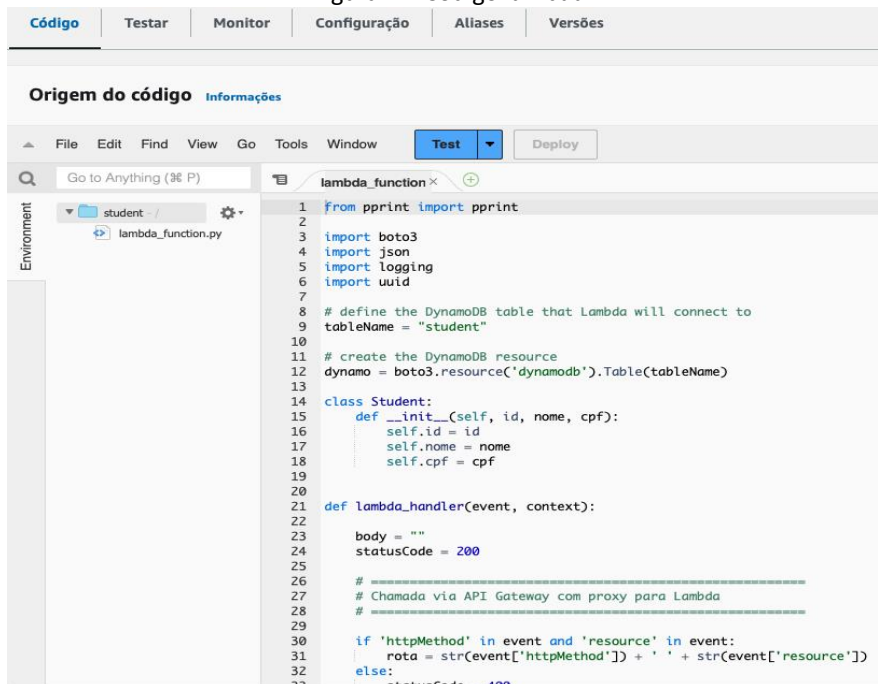
Figura 7 – Código lambda
