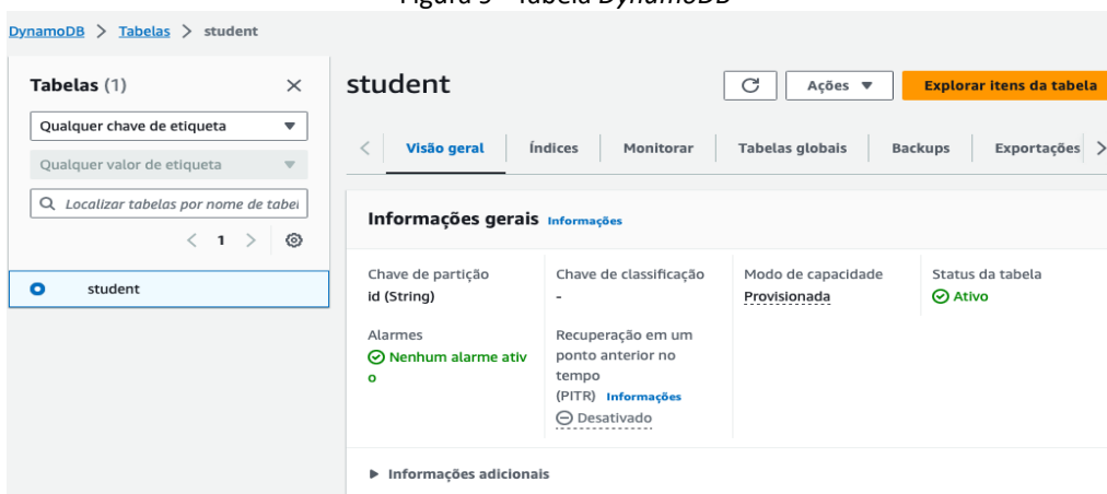
Figura 9 - Tabela DynamoDB
